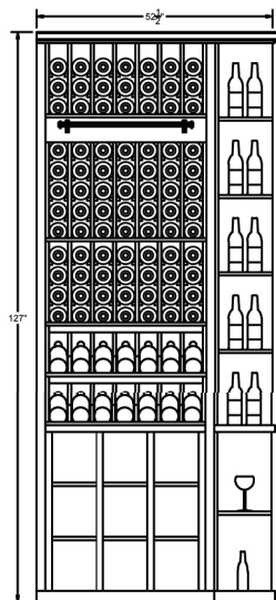
ELEVATION -D-
